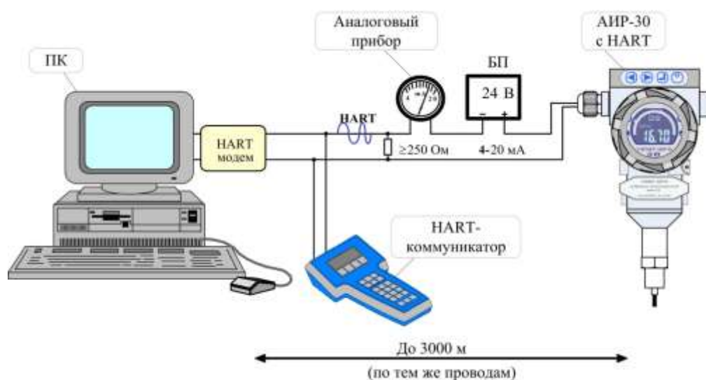
Схема подключения АИР-30 с HART-протоколом
