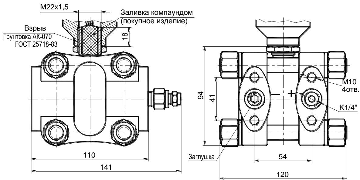
Чертеж средств взрывозащиты.
