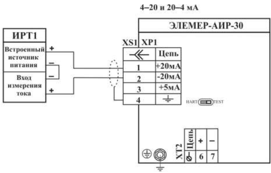
Схема электрическая подключений токовых цепей ЭЛЕМЕР-АИР-30 к различным приборам с разъёмами ШР14, ШР22 (цепи каналов сигнализации не показаны)
