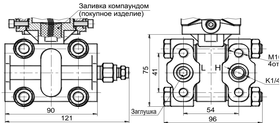
Чертеж средств взрывозащиты.
