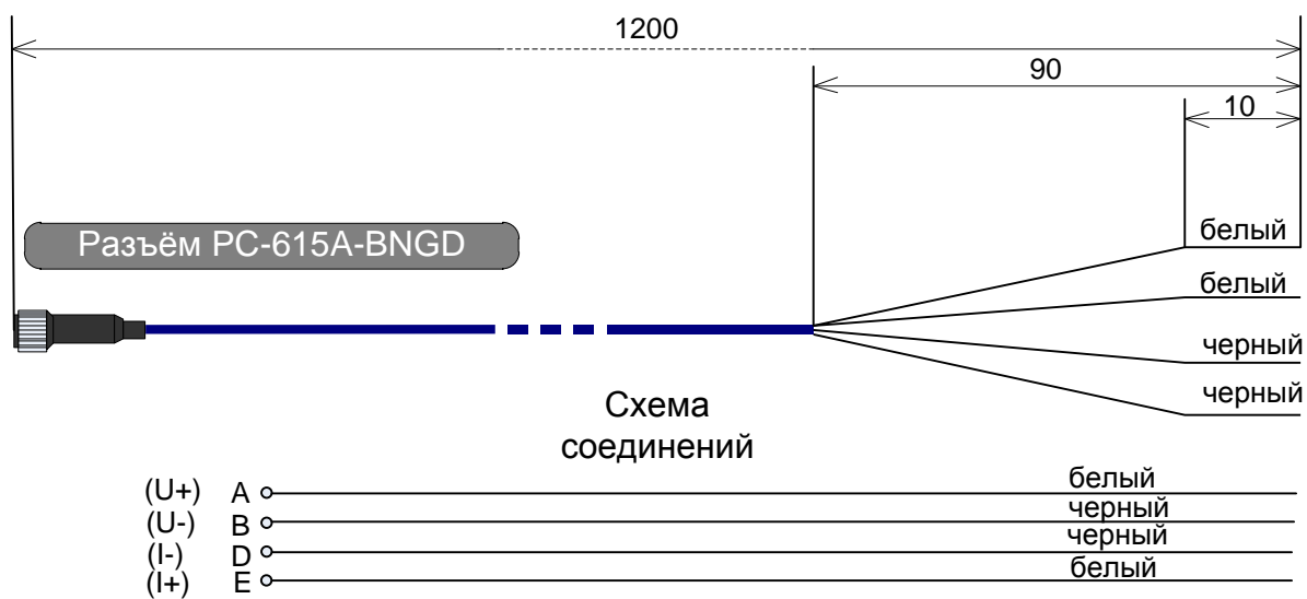
Рисунок А.4 – Кабель измерительный
