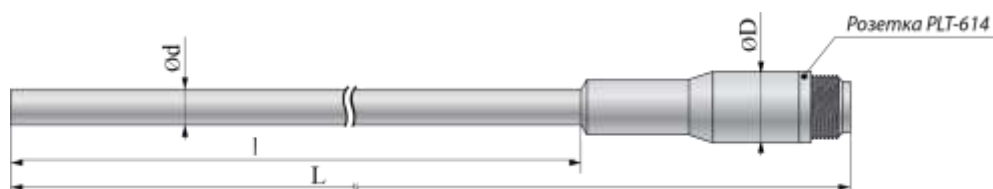
Рисунок А.1 - ПТСВ-1, ПТСВ-3, ПТСВ-4, ПТСВ-5
