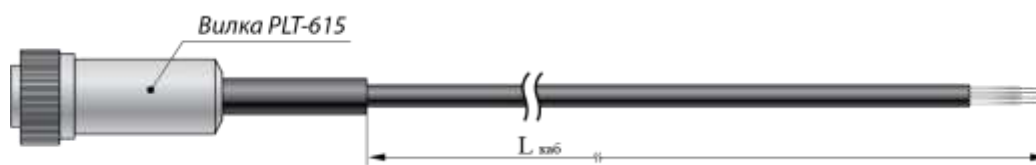
Рисунок А.5 - Кабель измерительный КИ-ТЦЭ
