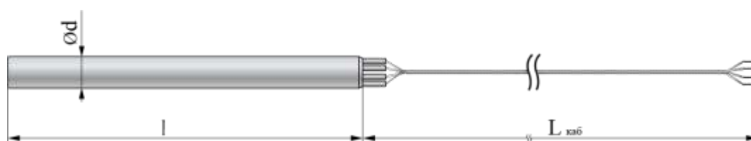
Рисунок А.2- ПТСВ-2
