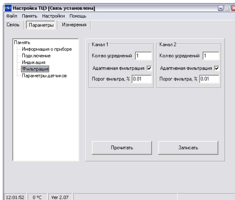
Рисунок 2.2- Закладка «Фильтрация»
