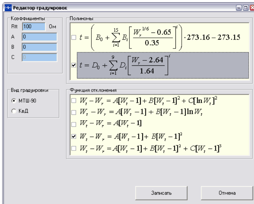
Рисунок 3.7
