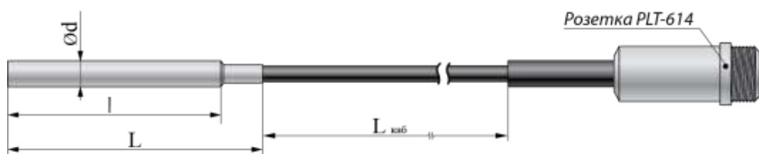
Рисунок А.3- ПТСВ-2К
