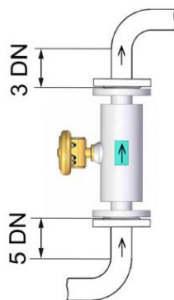
Двухлучевой датчик
