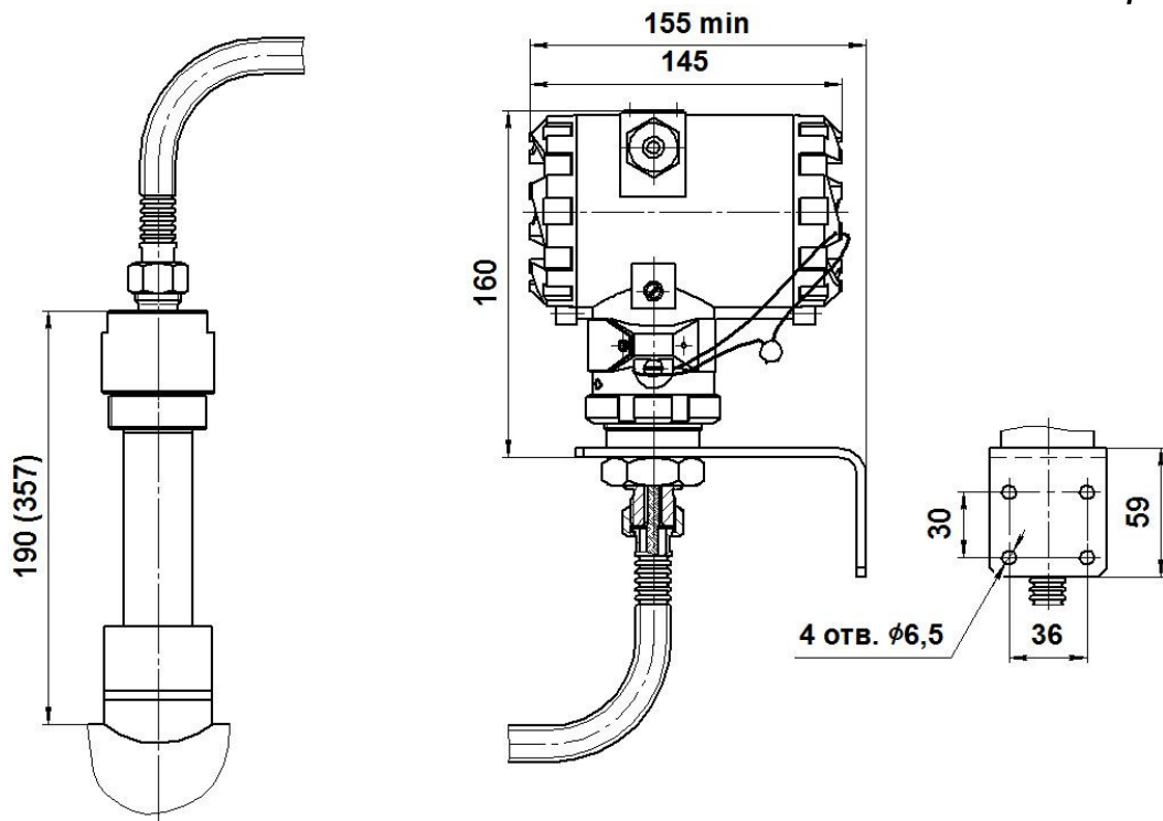
Рисунок В.11 - Размеры преобразователей дистанционного исполнения. Остальные размеры см. Рис. В.3 - В.8
