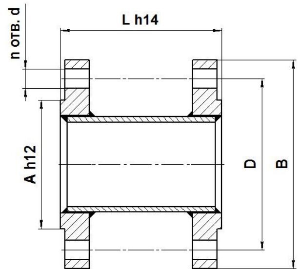
Рисунок В.11 - Размеры преобразователей дистанционного исполнения. Остальные размеры см. Рис. В.3 - В.8
