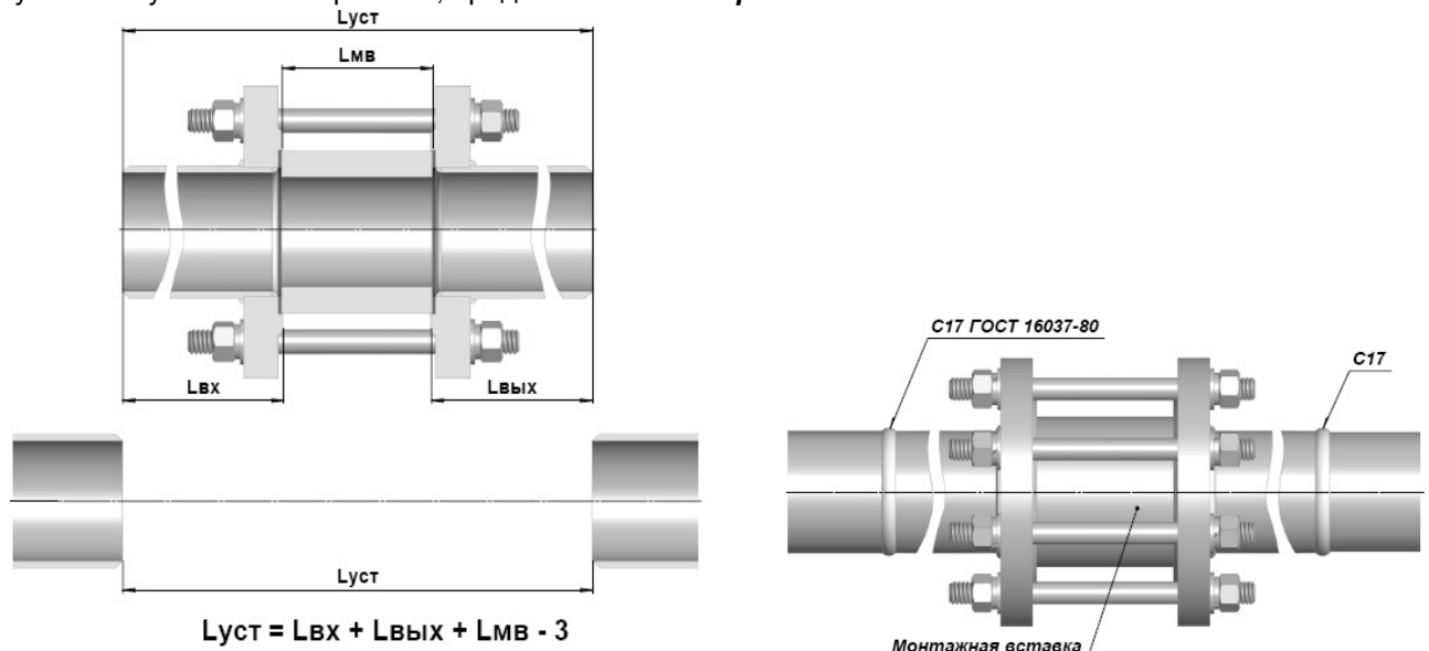
Рисунок 2.11 - Установка вставки с прямыми участками
