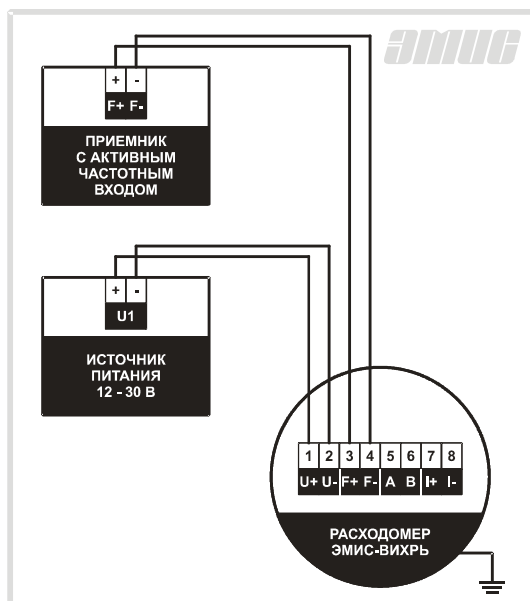
Рисунок Б.2 - Схема подключения к прибору с активным частотным входом
