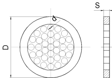
Рисунок 2.9 - Выпрямитель потока
