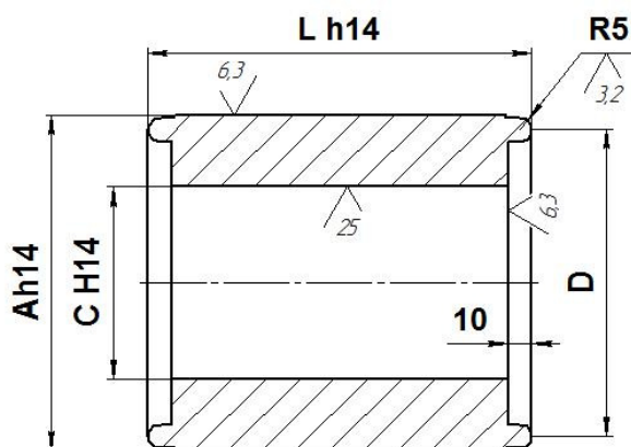
Рисунок В.11 – Размеры монтажных вставок см. Рис. В.3 - В.6
