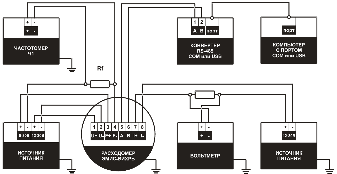
Рисунок Б.9 – Схема подключения при поверке проливным методом
