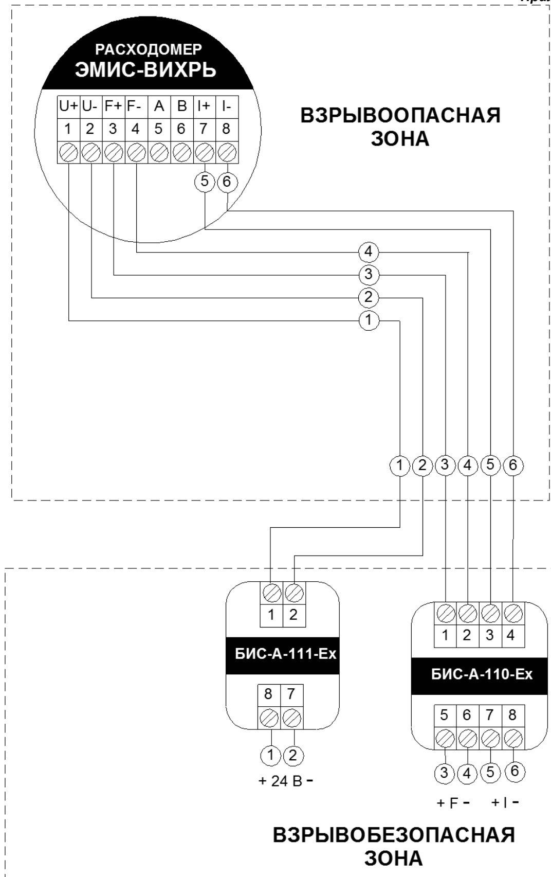
Рисунок Б.8 –Схема подключения преобразователей взрывозащищенного исполнения ExB через барьеры искрозащиты с использованием частотного и токового выходных сигналов (для приемников с активными входами)
