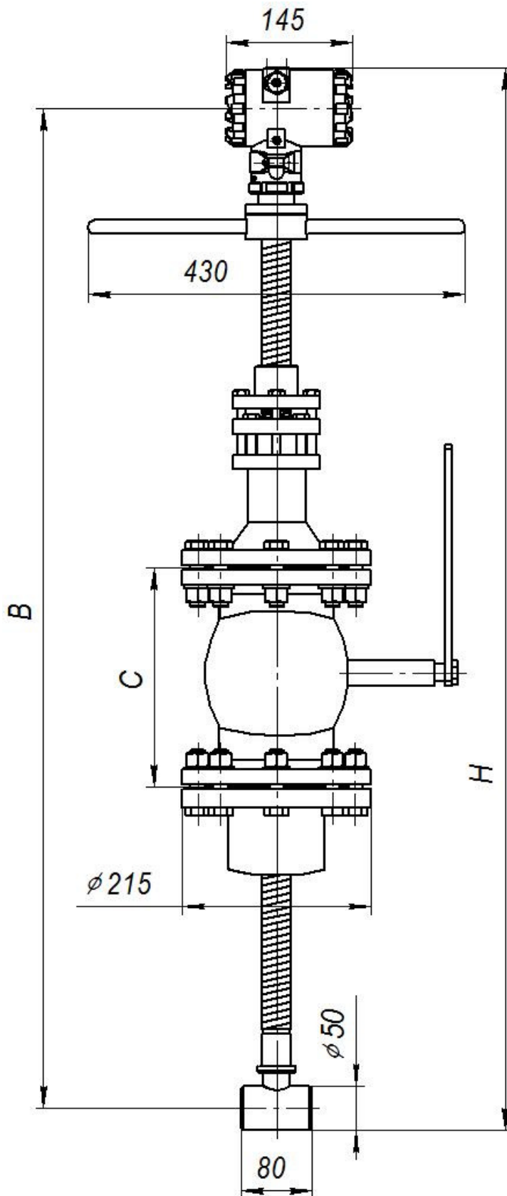
Рисунок В.9 - Размеры погружного преобразователя на давление 1,6 МПа
