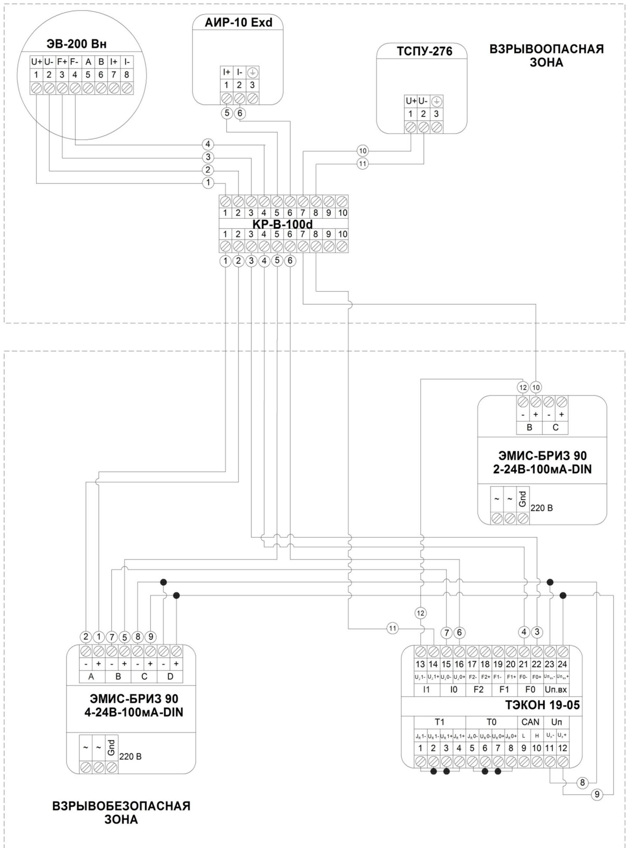
Схема 5. – Подключение узла типа Exd во взрывоопасной зоне с взрывозащищенным датчиком температуры
