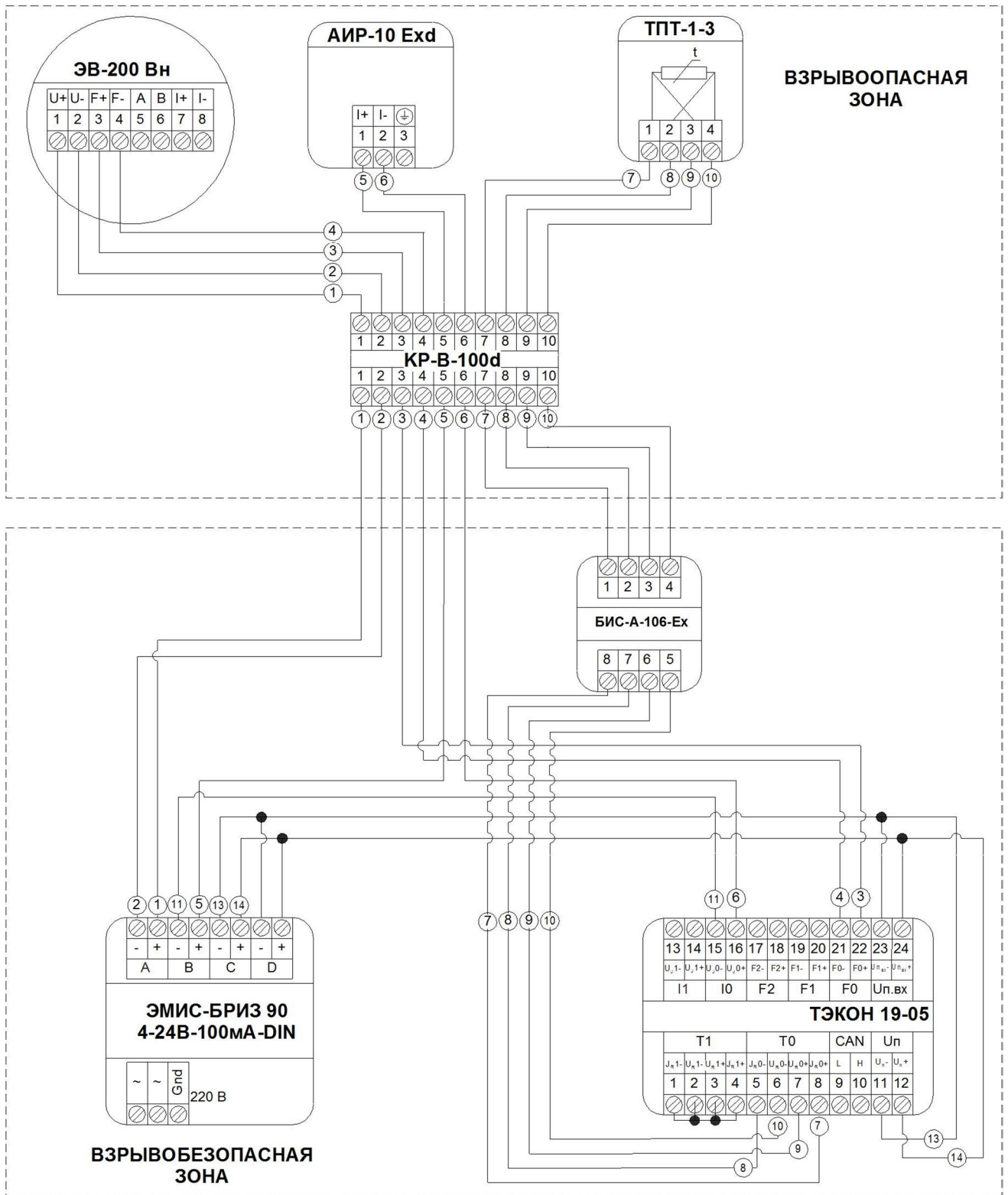
Схема 3. – Подключение узла типа Exd во взрывоопасной зоне с общепромышленным датчиком температуры
