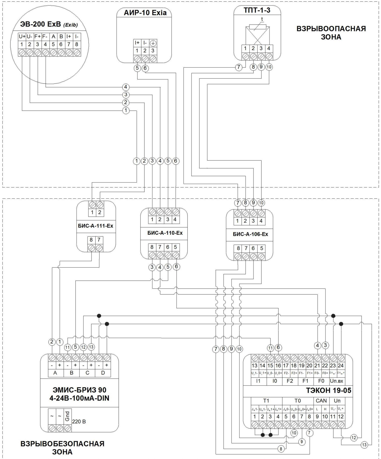
Схема 4. – Подключение узла типа Exib во взрывоопасной зоне с общепромышленным датчиком температуры
