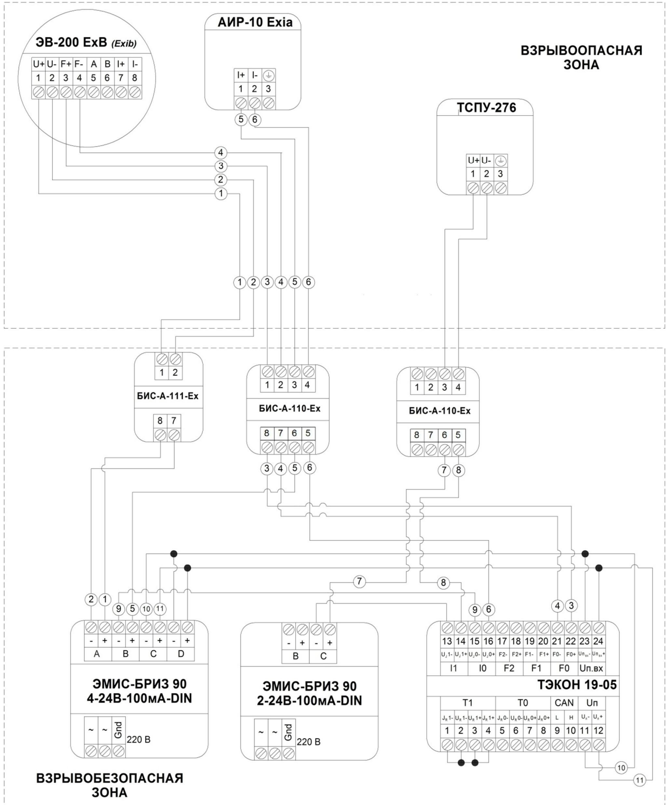
Схема 6. – Подключение узла типа Exib во взрывоопасной зоне с взрывозащищенным датчиком температуры
