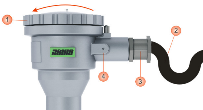
Рисунок 2.4 – Общие правила выполнения электрических подключений
