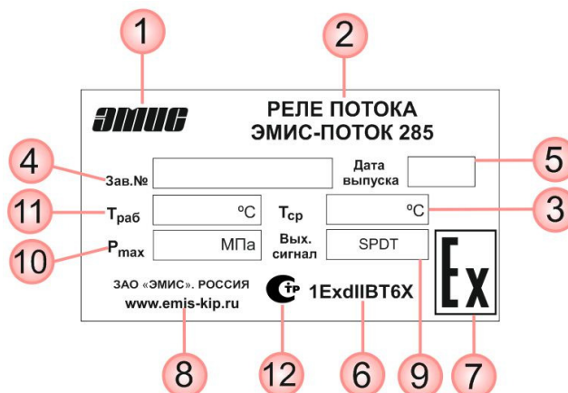
Рисунок 1.4 - Табличка реле потока
