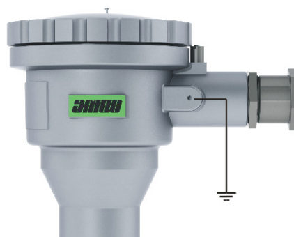
Рисунок 2.6 – Заземление реле потока
