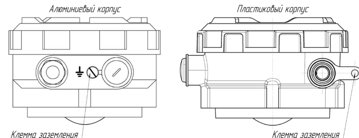
Рис. 5.2 Клемма заземления
