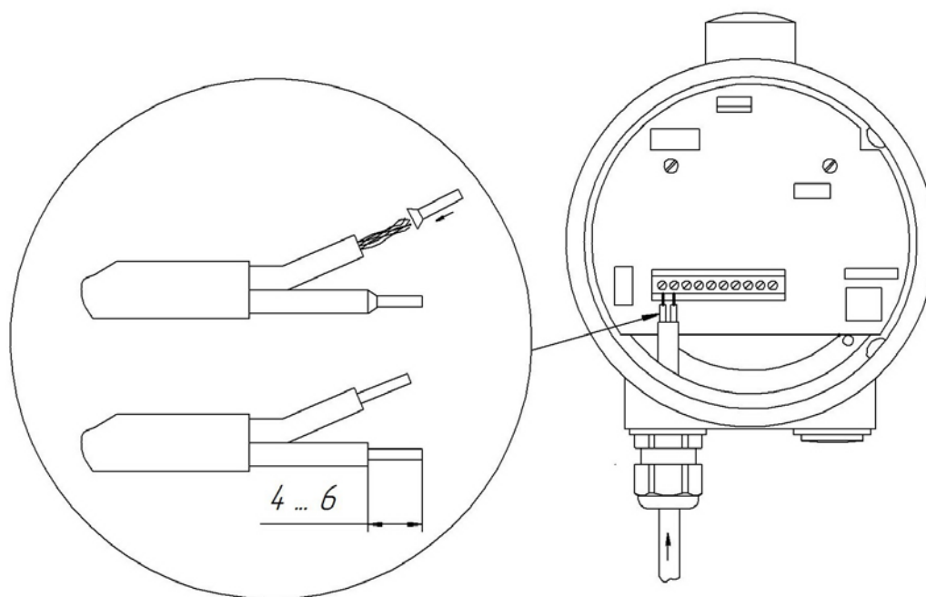
Рис. 5.9 Подключение уровнемера.
