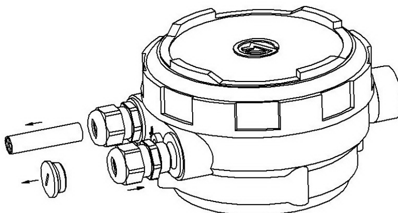
Рис. 5.8 Установка второго кабельного ввода
