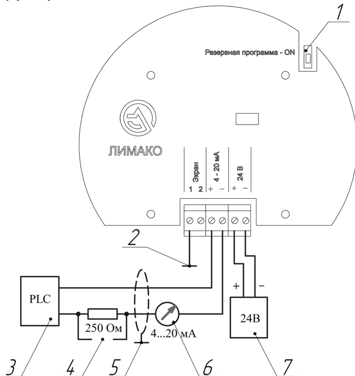
Рис. 5.5 Подключение уровнемера модификации УЛМ-31А1-НF-F-LC.
