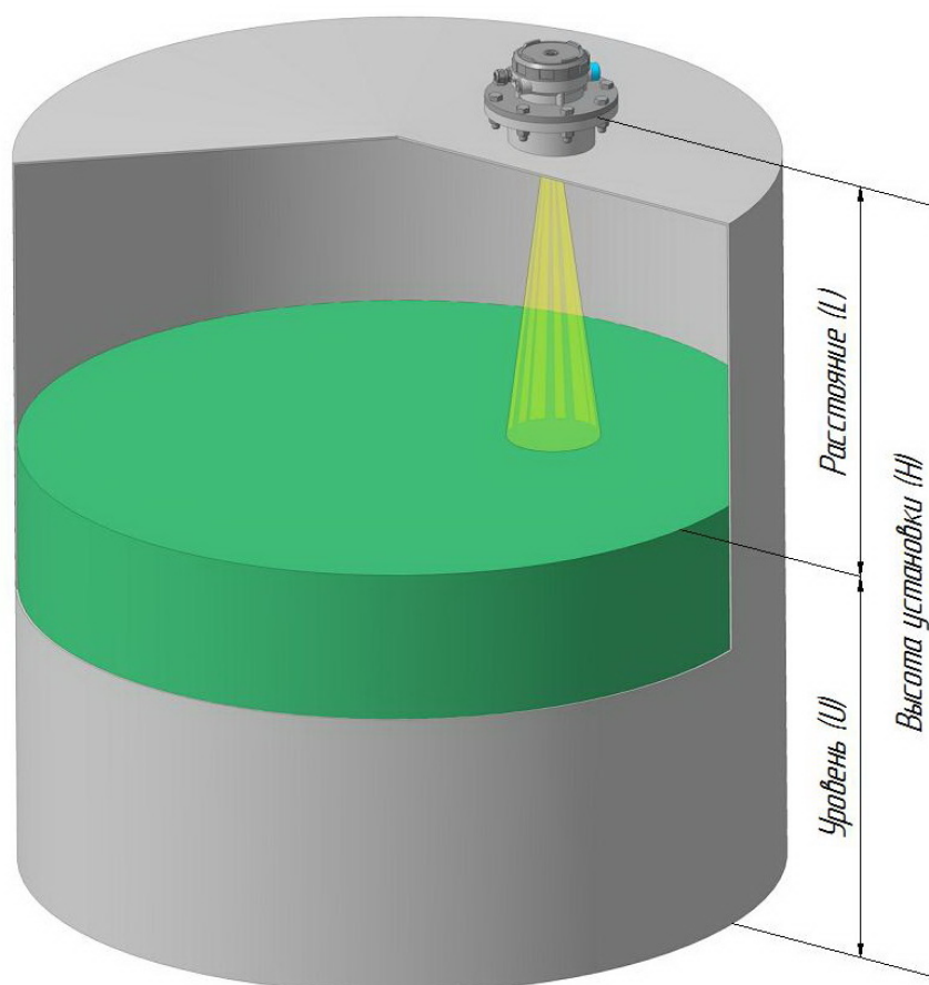
Рис. 3.6. Уровнемер на резервуаре.
