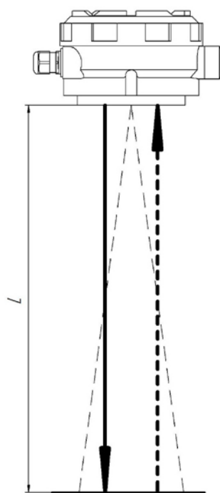
Рис. 3.7. Принцип измерения.
