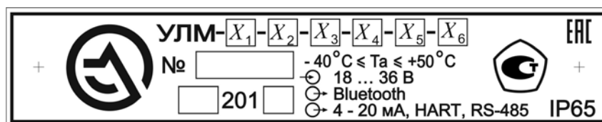
Рис. 3.5. Пример типового шильдика уровнемера.
