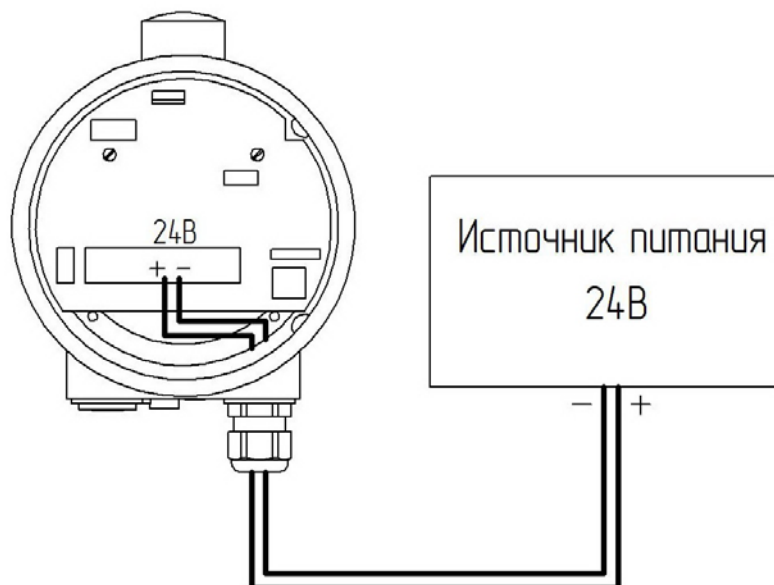
Рис. 5.6 Схема подключения уровнемера к ИП
