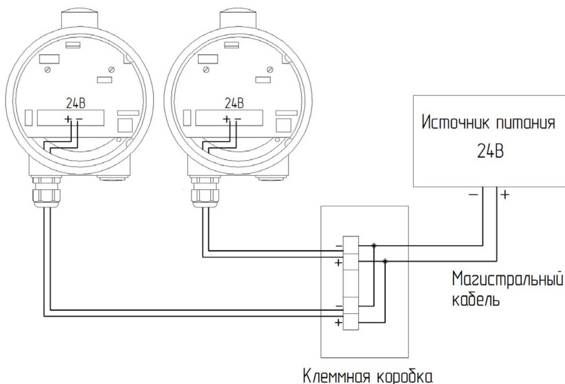
Рис. 5.7 Схема подключения уровнемеров к ИП с использованием клеммной коробки.
