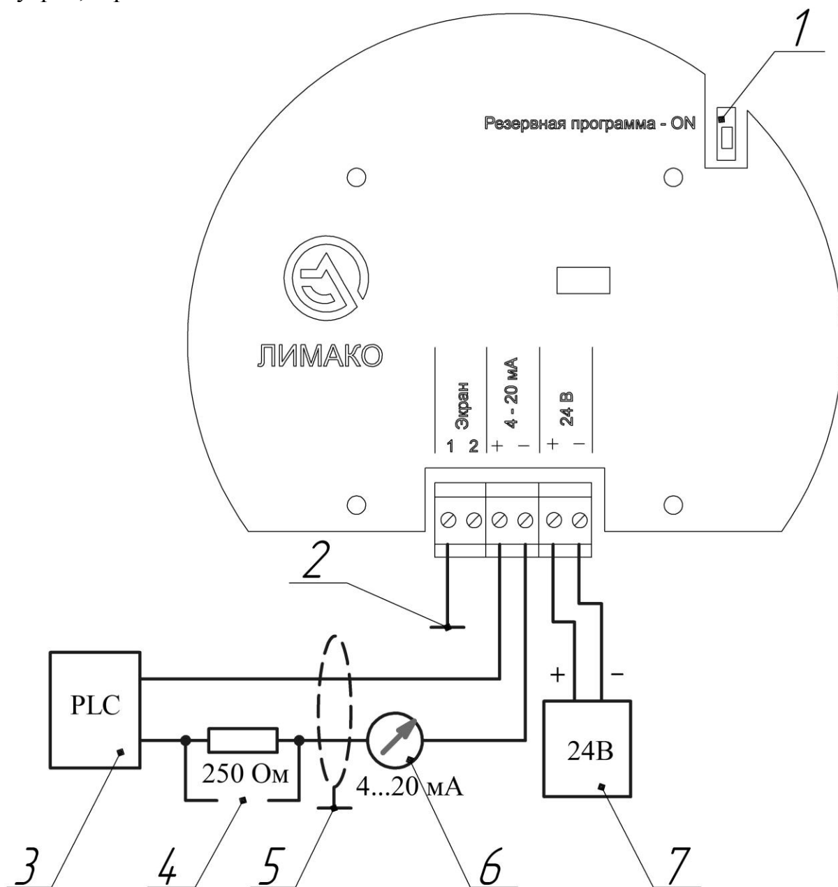
Рис. 5.4 Подключение уровнемера модификации УЛМ-31А1-НФ-Ф-ЛС.
