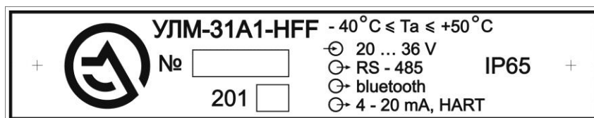
Рис. 3.8. Типовой шильдик УЛМ-31А1-НФ-F
