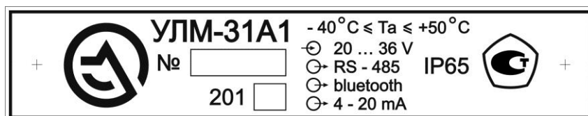
Рис. 3.6. Типовой шильдик УЛМ-31А1
