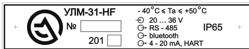
Рис. 3.5. Типовой шильдик УЛМ-31-НФ
