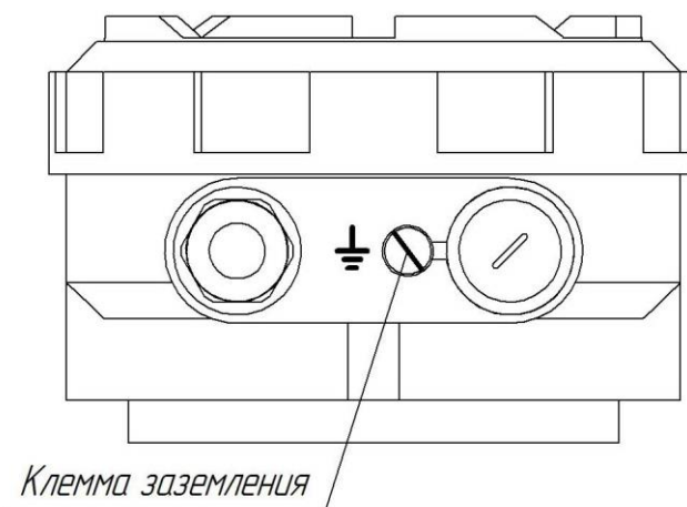
Рис. 5.2 Клемма заземления
